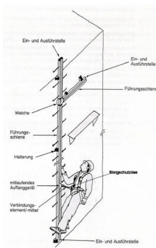
Bild 15: Beispiel für eine Steigschutzeinrichtung, bestehend aus einer vertikalen und einer horizontalen Führung (Übergang mit Weiche)
