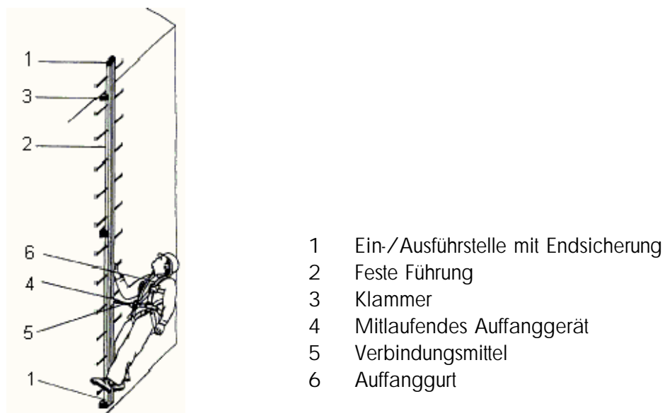
Bild 3: Skizze des Auffangsystems mit mitlaufendem Auffanggerät einschließlich fester Führung (Steigschutzeinrichtung)
