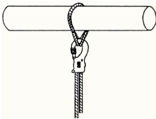
Bild 26: Richtiges Anschlagen: Zur Erhaltung der Funktionsfähigkeit des Falldämpfers wird ein Anschlagverbindungsmitel mit zwei Augen verwendet, welches über ein waagerechtes Tragelement gelegt wird; Einhaken des Karabinerhakens in die zwei Augen
