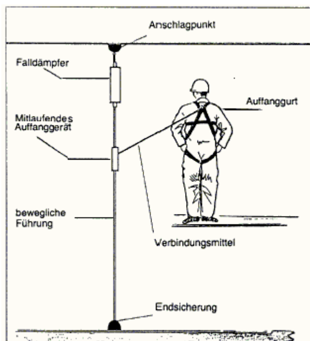
Bild 1: Systematische Darstellung des Auffangsystems:
