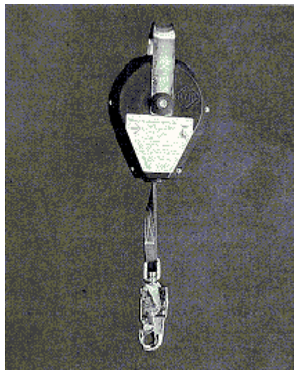
Bild 14: Höhsicherungsgerät mit einziehbarem Verbindungsmittel aus Gurtband
