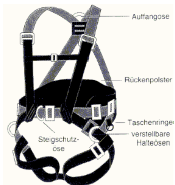
Bild 10: Auffanggurt mit rückseitiger Fangöse, zwei seitlichen Halteösen und einer vorderen Steigschutzöse; Rückenstütze bzw. Rückenpolster ist vorhanden
