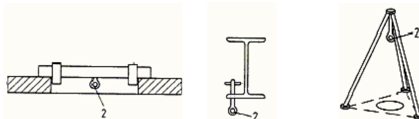
2 Anschlagpunkt
